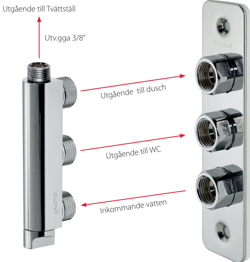
Ballofix® Minifördelare med inbyggd kulventil
