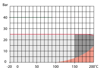
Svets × Svets - DN 40 - 150 - PN 25
