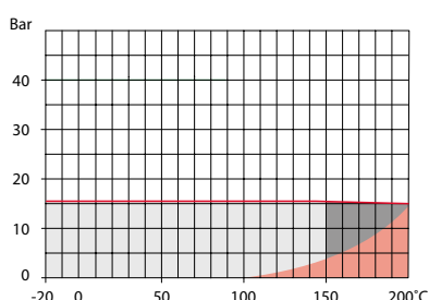
Flange × Flange - DN 40 - 150 - PN 16
