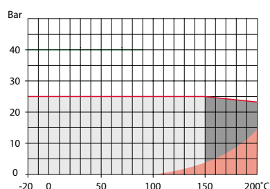
Flange × Flange - DN 40 - 150 - PN 25
